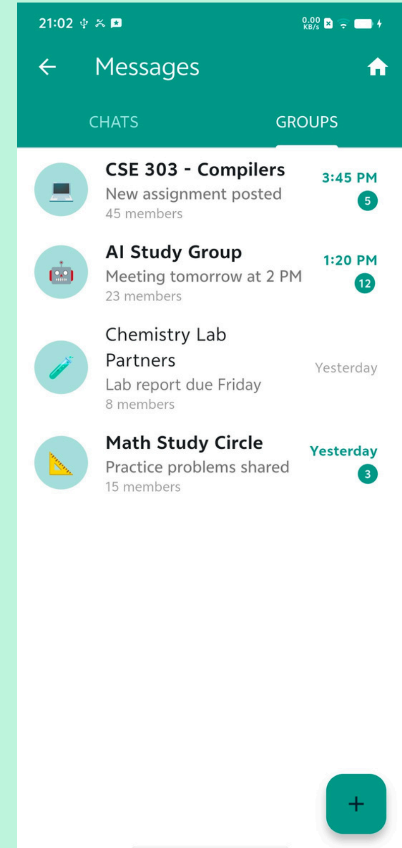
Message
