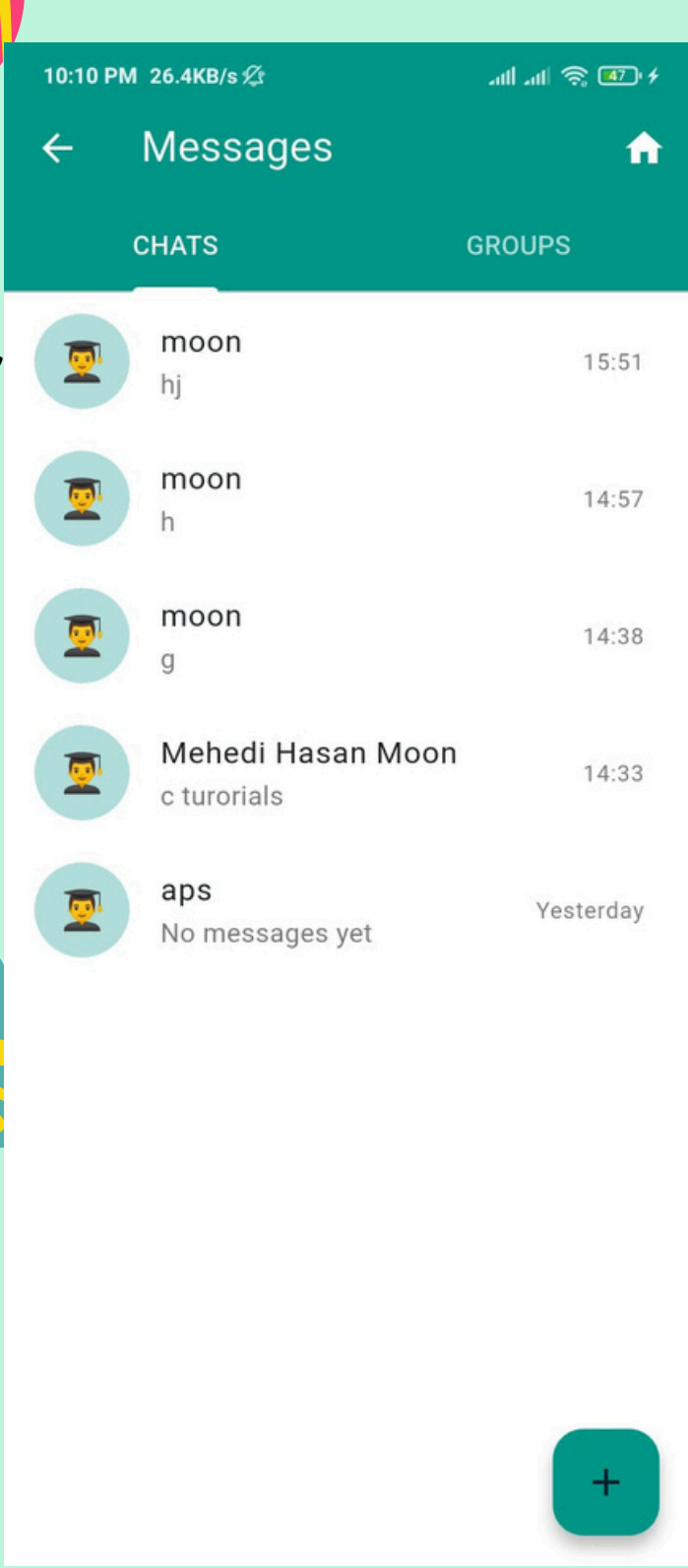
Chats
